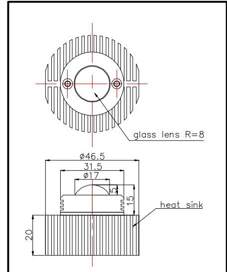
Outer dimension(Unit:mm)
