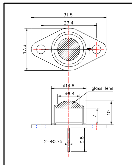
Outer dimension(Unit:mm)
