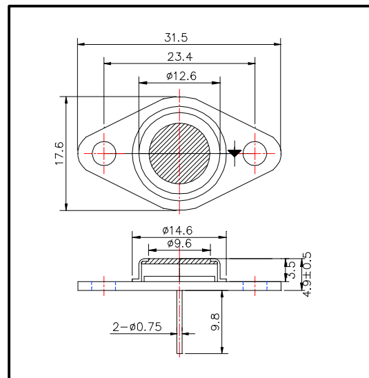
Outer dimension(Unit:mm)
