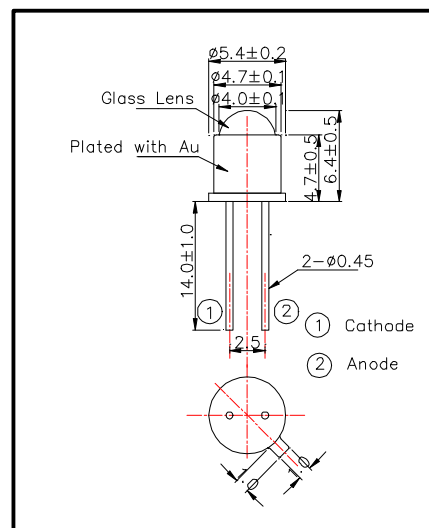
Outer dimension(Unit:mm)
