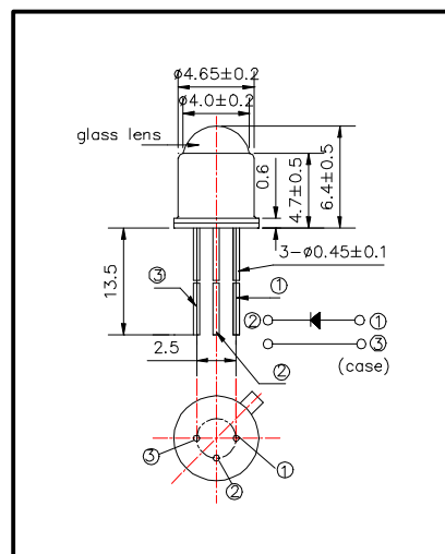
Outer dimension(Unit:mm)
