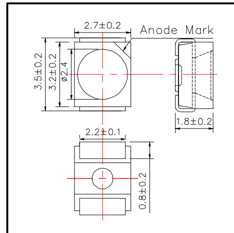
Outer dimension(Unit:mm)
